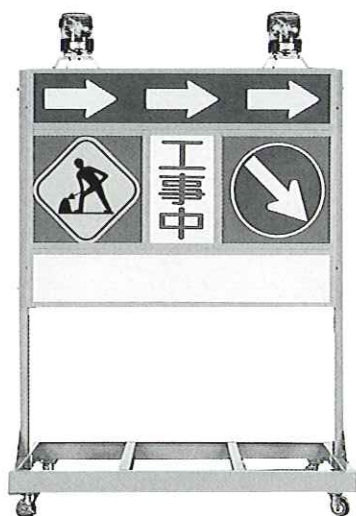
GE-51 サイズ：W1,650×H2,250×D1,200mm 総重量：約85kg
