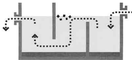
断面図
